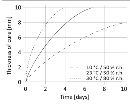
Діаграма 1: Швидкість полімеризації SikaTack® Panel-50
