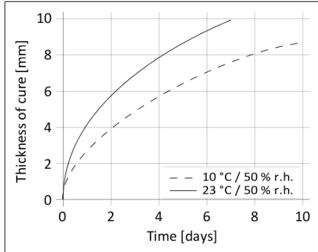
แผนภาพที่ 1: อัตราการแห้งตัวของ Sikaflex®-295 UV
