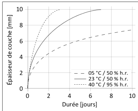
Diagramme 1: Vitesse de polymérisation du Sikasil® WS-605 S
