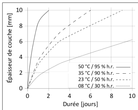
Diagramme 1: Vitesse de durcissement de Sikasil® AS-70
