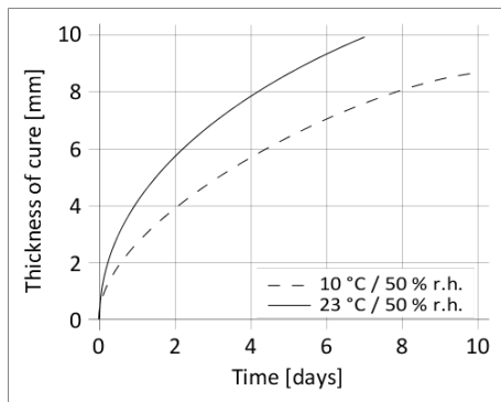
Graf 1: Rýchlosť vytvrdzovania Sikaflex®-295 UV
