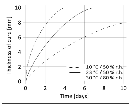
Graf 1: Rýchlosť vytvrdzovania SikaTack® Panel-50
