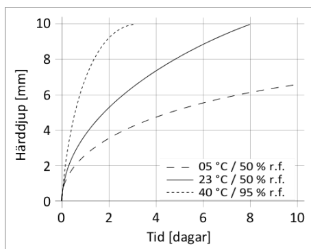
Diagram 1: Härdningshastighet hos Sikasil® WS-305 EU
