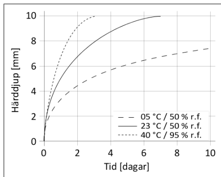
Diagram 1: Härdningshastighet Sikasil® WS-605 S
