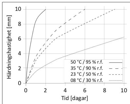
Diagram 1: Härdningshastighet Sikasil® WT-40
