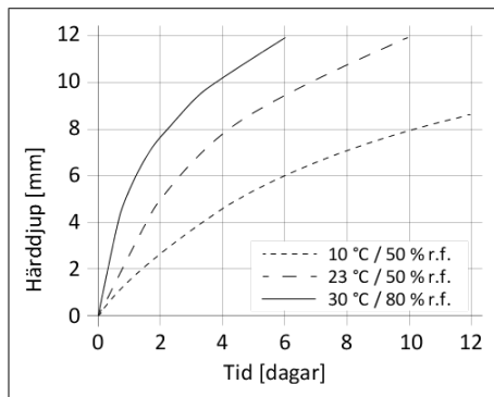
Diagram 1: Härdningshastighet Sikaflex®-268
