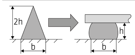
Figura 1: Configuração recomendada do cordão
