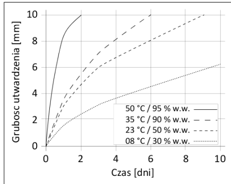
Wykres 1: Szybkość utwardzania Sikasil® WT-40
