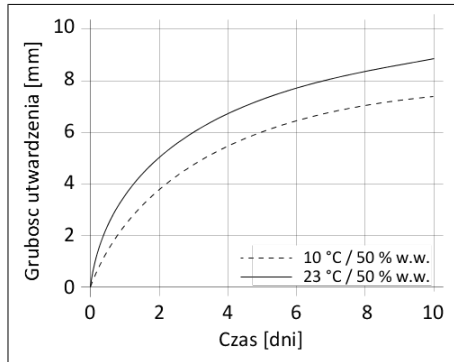
Wykres 1: Szybkość utwardzania Sikaflex®-292i
