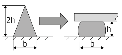
Figure 1: Anbefalt utforming av limstreng
