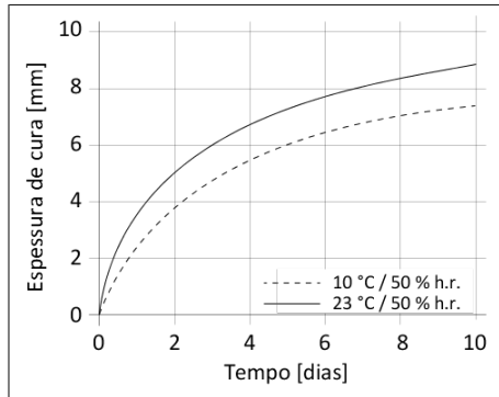
Diagrama 1: Velocidade de cura do Sikaflex®-292i
