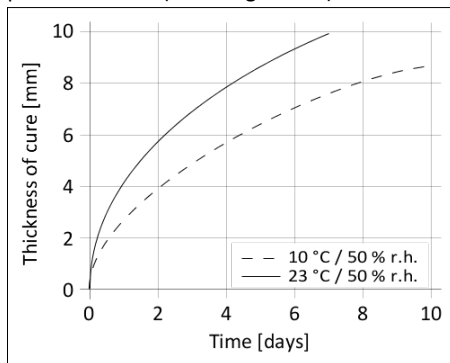
Diagramma 1: Velocità di indurimento per SikaTack® MOVE Transportation
