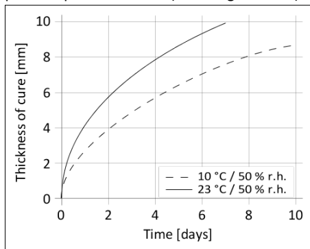
Diagramma 1: Velocità di indurimento per SikaTack® PRO
