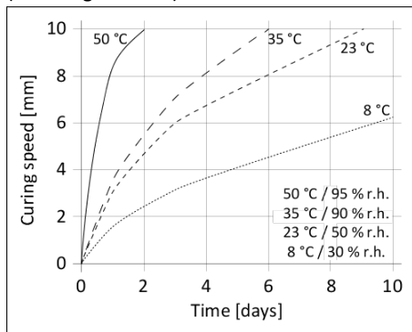
Diagramma 1: velocità di indurimento Sikasil® IG-16
