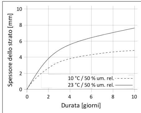
Grafico 1: Velocità di indurimento per Sikaflex®-522
