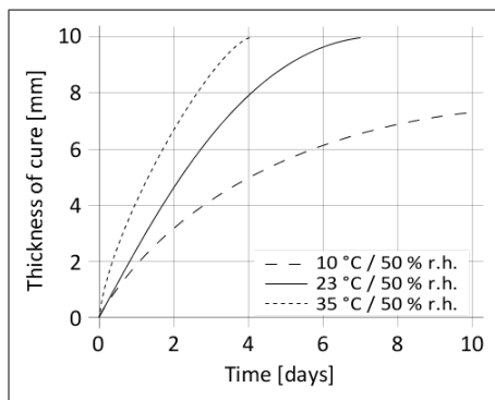
Diagramma: velocità di indurimento di Sikaflex®-276 PC-2
