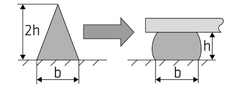
Εικόνα 1: Συνιστώμενος τρόπος διαμόρφωσης τριγωνικού κορδονιού
