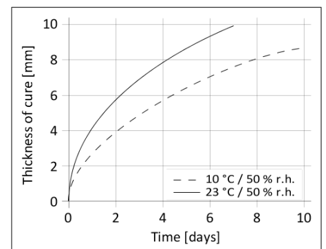
Διάγραμμα 1: Ταχύτητα ωρίμανσης Sikaflex®-296
