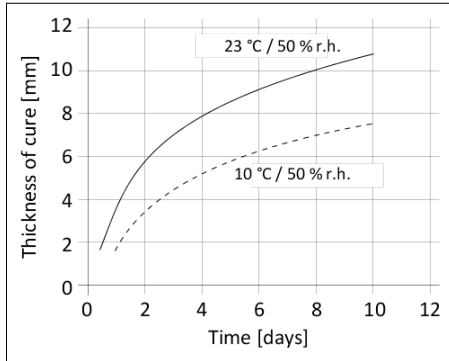
Διάγραμμα 1: Αντίδραση ωρίμανσης για το Sikaflex®-291i.
