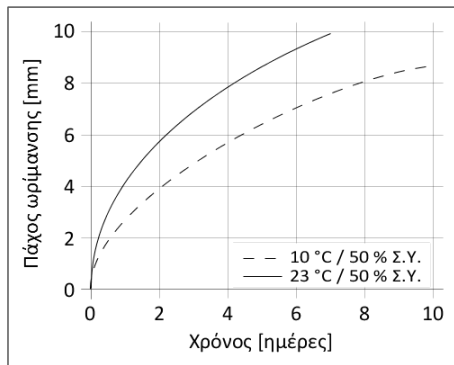
Διάγραμμα 1: Ταχύτητα ωρίμανσης του Sikaflex®-290 DC PRO
