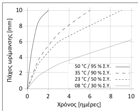
Διάγραμμα 1: Ταχύτητα ωρίμανσης Sikasil® WT-40
