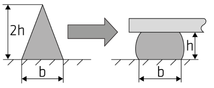
Σχήμα 1: Συμπίεση κορδονιού συγκολλητικού στο τελικό μέγεθος
