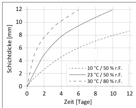
Diagramm 1: Durchhärtengeschwindigkeit Sikaflex®-250 PC
