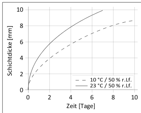
Diagramm 1: Durchhärtengeschwindigkeit von Sikaflex®-223
