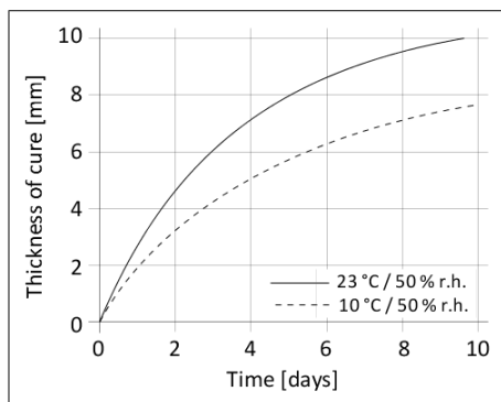
Graf 1: Rychlost vytvrzování Sikaflex®-515
