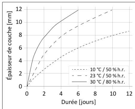
Diagramme 1: Vitesse de durcissement de Sikaflex®-268
