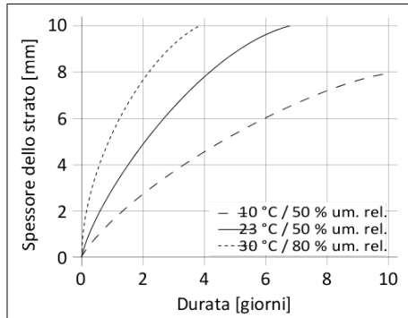
Diagramma 1: velocità di polimerizzazione di SikaTack® Panel-50
