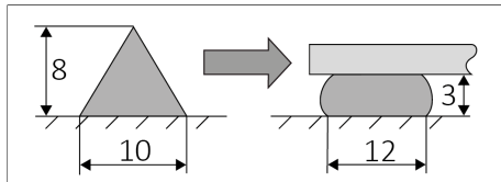
Figura 1: applicazione raccomandata dell'adesivo
