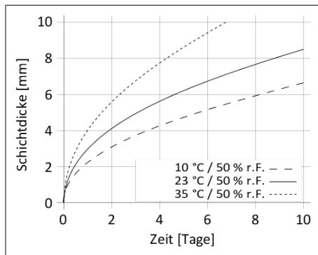
Diagramm 1: Durchhärtengeschwindigkeit Sikaflex®-554
