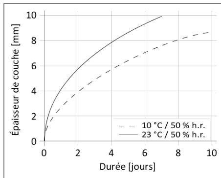
Diagramme 1: Vitesse de durcissement de SikaTack® PRO
