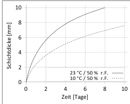
Diagramm 1: Durchhärtageschwindigkeit von Sikaflex®-291i
