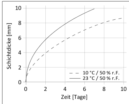
Diagramm 1: Durchhärtengeschwindigkeit SikaTack® MOVE Transportation
