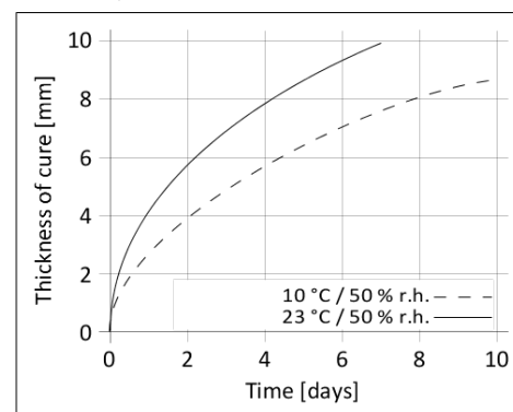
Schéma 1 : Vitesse de mûrissement du Sikaflex® SOLO
