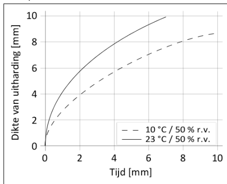
Schema 1: Uithardingsnelheid SikaTack® PRO
