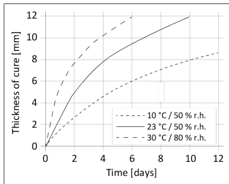
Diagramm 1: Durchhärteschwindigkeit Sikaflex®-252
