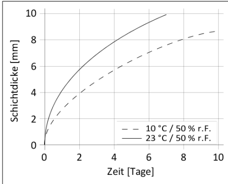
Diagramm 1: Durchhärtengeschwindigkeit für Sikaflex®-290 DC PRO
