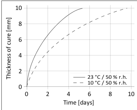
Diagramm 1: Durchhärtegeschwindigkeit Sikaflex®-298
